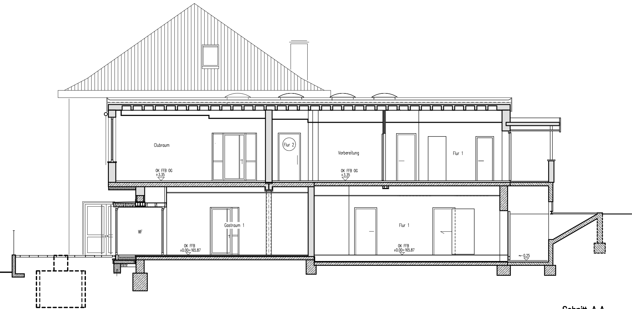
Schnitt A-A
