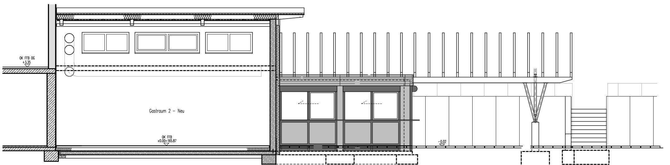
Schnitt C-C
